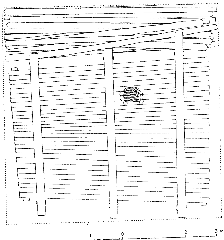
Р и с. 2. План могилы на уровне потолка.
